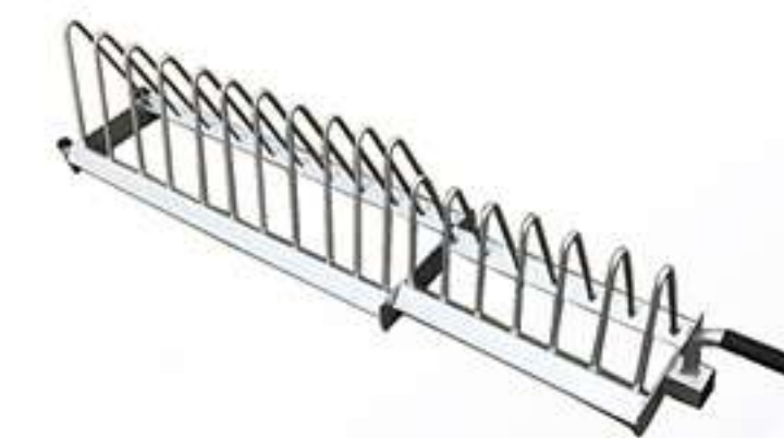
HJ-00234 杠铃片架 Weight Plates Rack 占地面积/Space: L-840 W-840 H-1260mm 体积/CBM: 0.05m³ 毛重/G.W.: 30KG 起订量/MOQ: 10PCS 参考价/RMB: 1920/PCS
