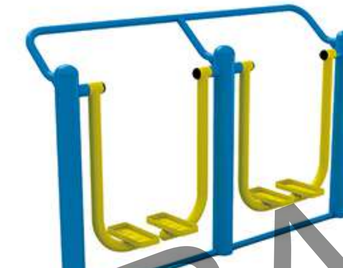
HJ-W021 双人太空漫步机 Double People Air Walker SPEC:2100*560*1560MM RMB: 5400/PCS
